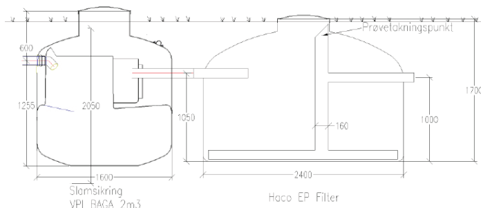
Målsatt skisse
